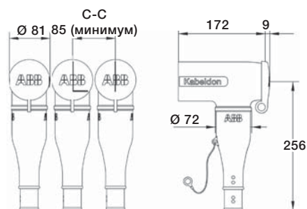
CSE-A 630 A, 12-24 кВ, размеры 1-2.
