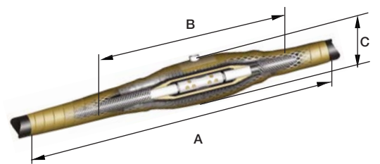
SOJ с внешней оболочкой с армированием из литьевой смолы
