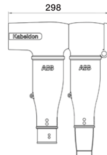
CSE-A, размеры 1-2 + CSAP-A CSE-A, размер 3 + CSAP-A
